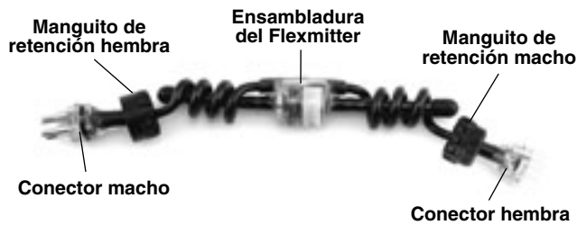
Figura 6 – Flexmitter
