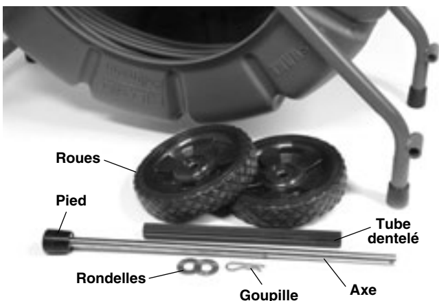
Figure 11 – Composants de l'ensemble de roulement
